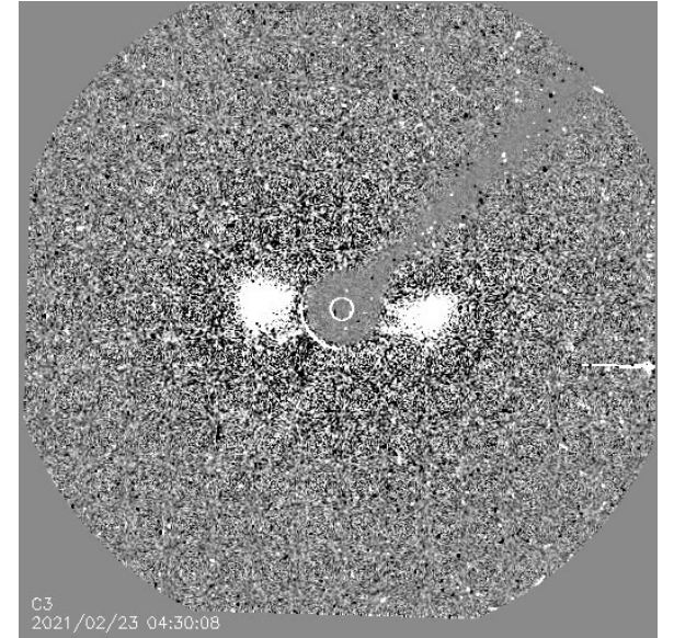
LASCO C3
