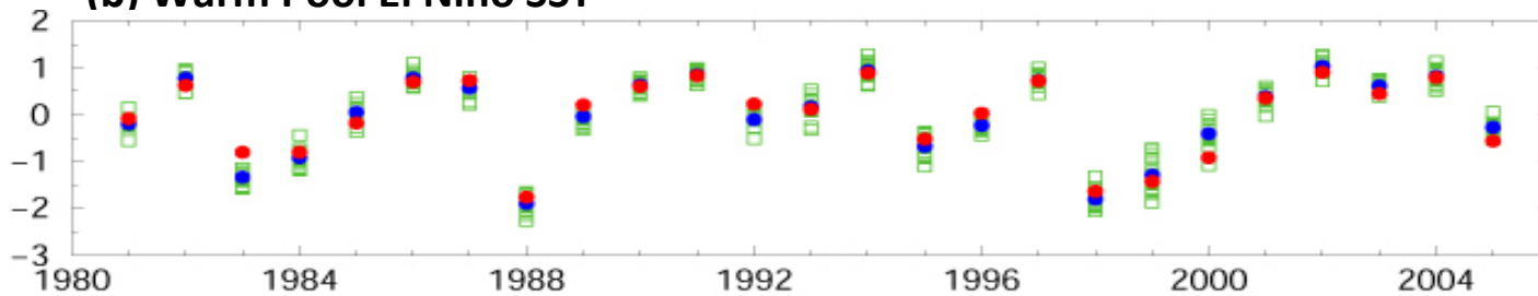
(c) Cold Tongue El Niño SST
